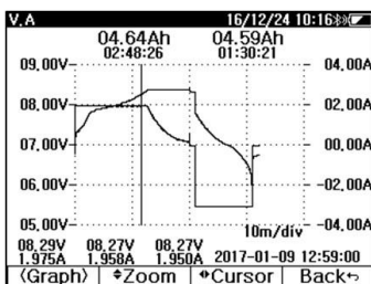
Wywołanie testu ładowania/rozładowania – wykres
