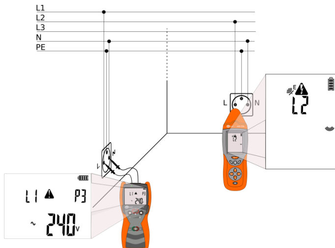
Rys. 34 Identyfikacja fazy.
