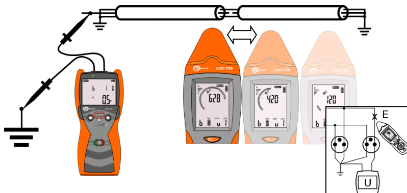
Rys. 26 Lokalizacja przerwy.
