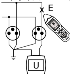
Rys. 8 Schemat trybu napięciowego.
