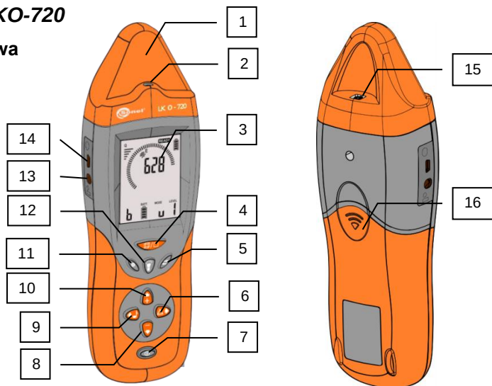
Rys. 3 Odbiornik.
