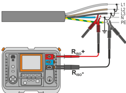
Rys. 4.1. Pomiar kabla nieekranowanego
