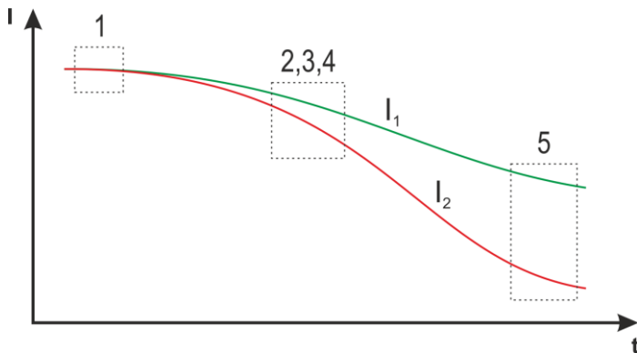
Wykres 4.3. Wpływ cech materiału na krzywe PDC.
