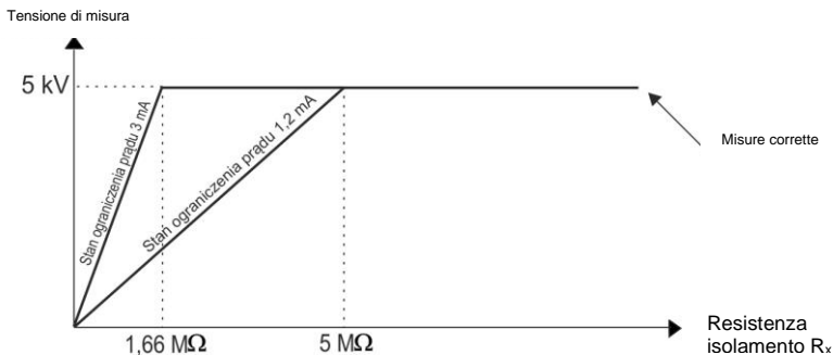
La tensione di prova effettiva in funzione della resistenza di isolamento misurata R_x (per la tensione di prova massima)
