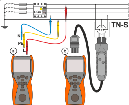
Medición en el circuito TN-S
