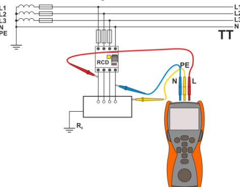
Medición en el circuito TT
