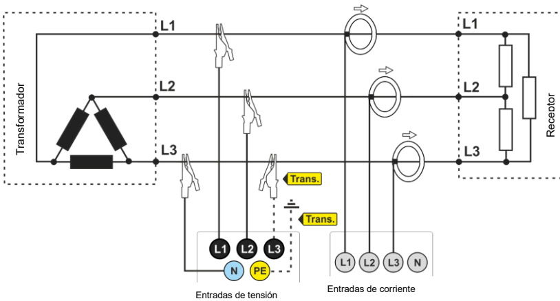
Fig. 20. Esquema de conexión – sistema trifásico tipo triángulo.
