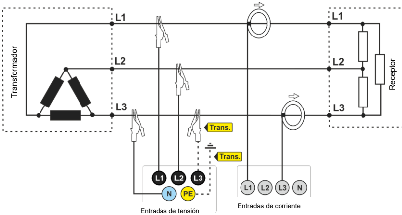
Fig. 21. Esquema de conexión – sistema trifásico tipo triángulo (medición de corrientes mediante el método de Aron).
