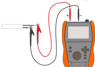
Medición R ISO estándar
