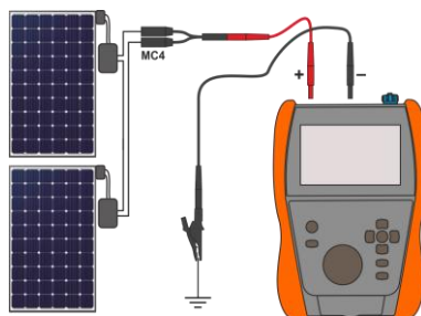
Medición R ISO en instalaciones fotovoltaicas equipadas con optimizadores
