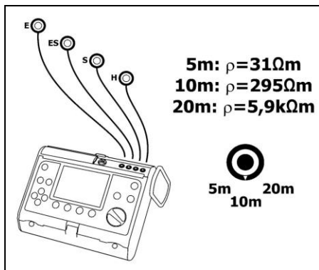
Fig. 15. Conexión del medidor.
