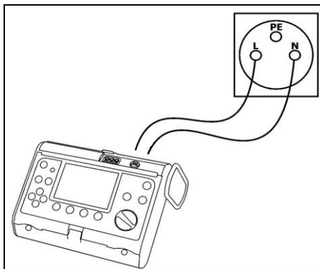
Fig. 18. Conexión del medidor
