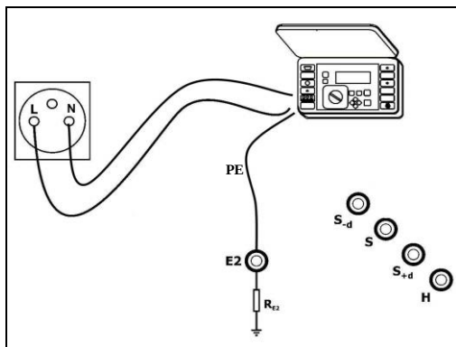
Fig.14. Conexión del medidor.
