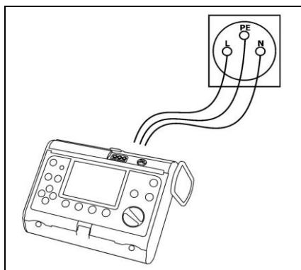
Fig.6. Conexión del medidor.
