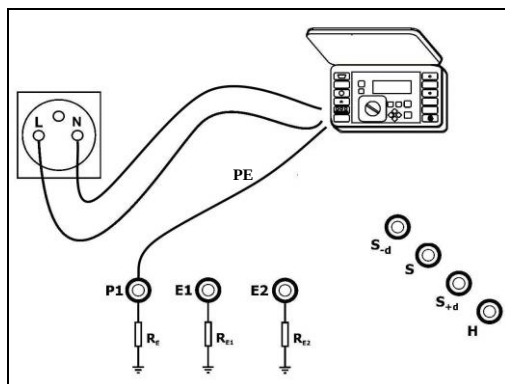
Fig. 12. Conexión del medidor.
