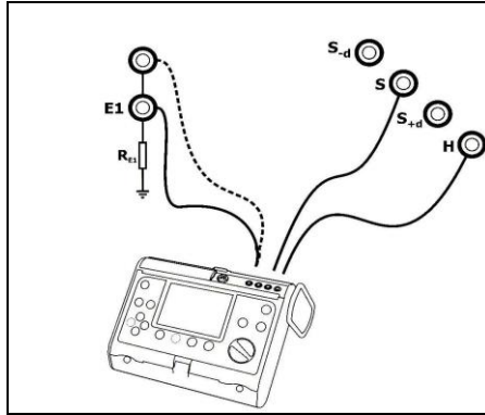
Fig.8. Conexión del medidor.
