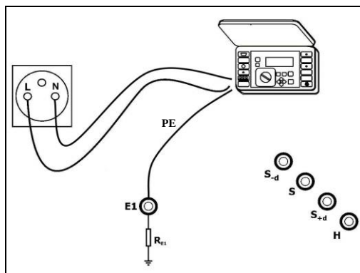
Fig.13. Conexión del medidor.
