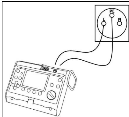
Fig. 19 Conexión del medidor.
