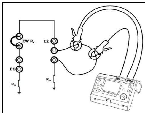
Fig.11. Conexión del medidor.
