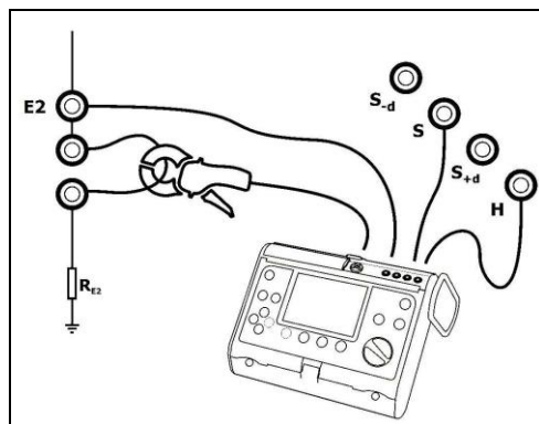
Fig. 10. Conexión del medidor.
