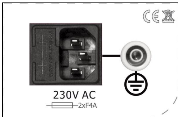
Fig.20. Colocación de los fusibles.
