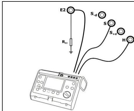
Fig.9. Conexión del medidor.
