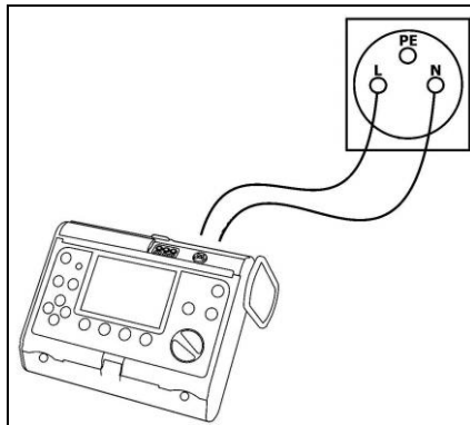
Fig.5. Conexión del medidor.
