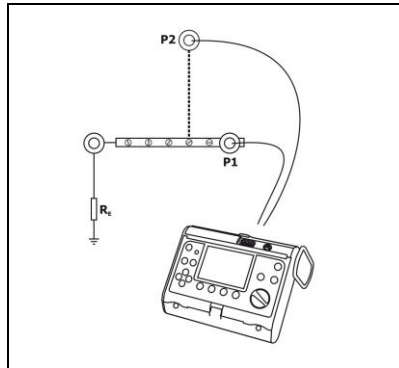
Fig. 16. Conexión del medidor.
