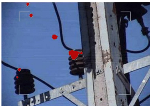
Rys. 9,10. Wyladowanie koronowe i jego skutki.
