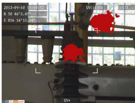
Rys. 3.4. Wyładowania koronowe w warunkach laboratoryjnych.
