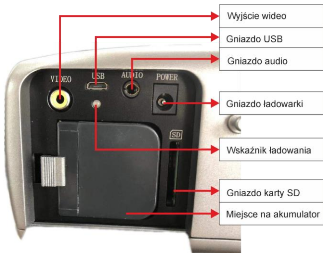
Rys. 15. Rozmieszczenie gniazd pod osłoną.
