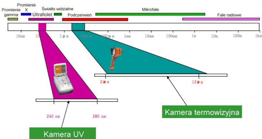
Rys. 1. Fale elektromagnetyczne różnej długości.
