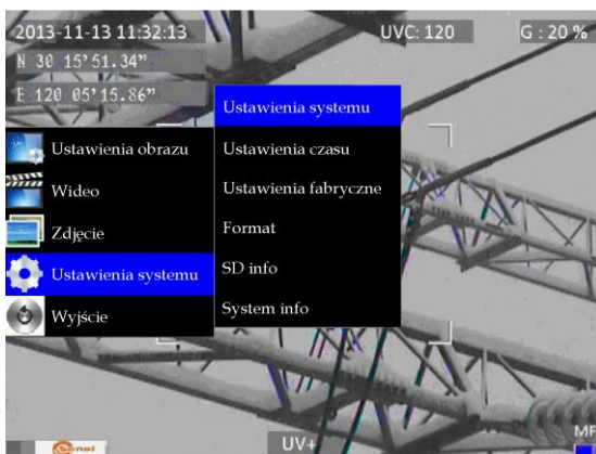
Rys. 20. Menu system.
